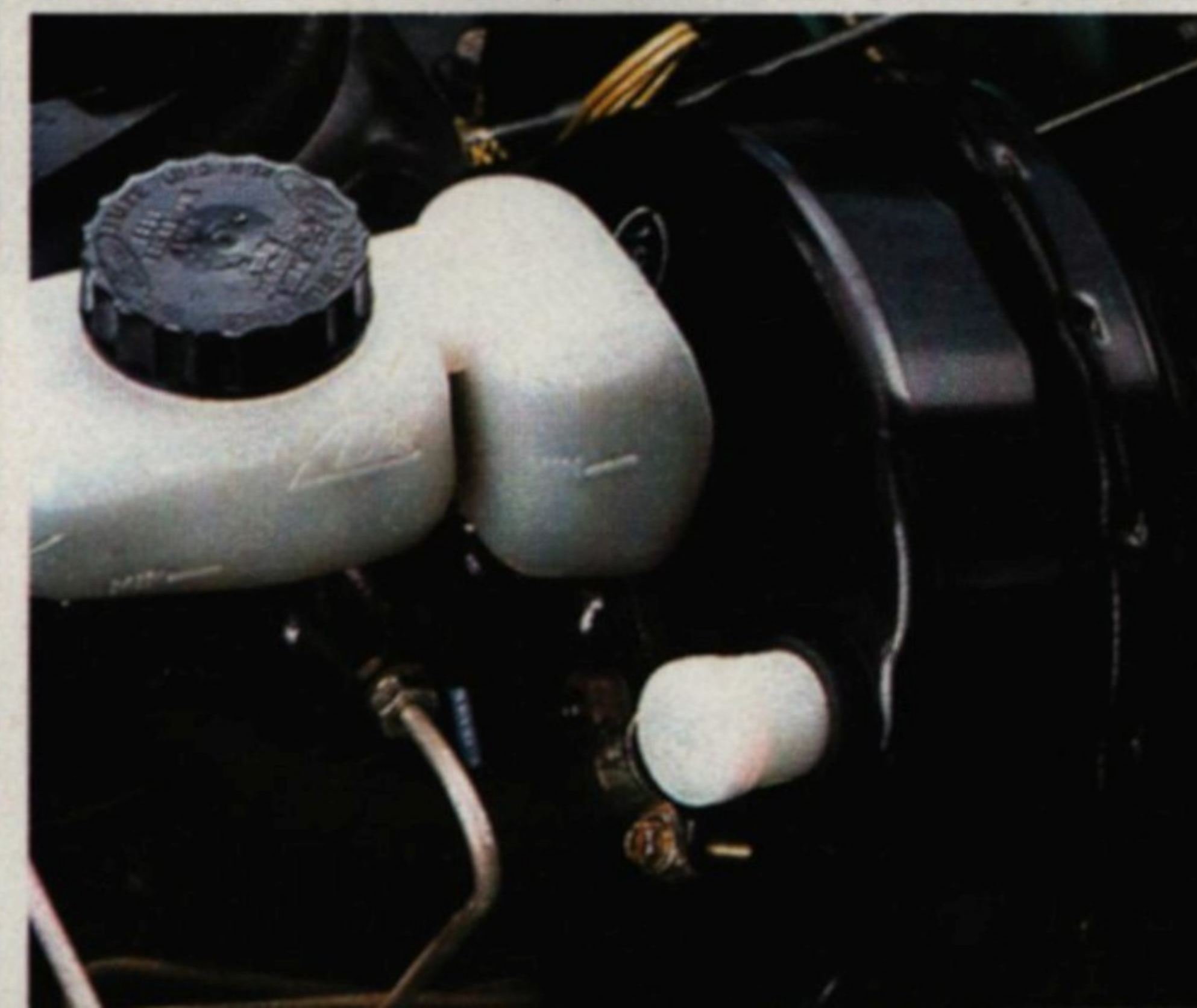
Stahl-Gürtelreifen ▲ ▼ Bremskraftverstärker und Scheibenbremsen vorn ▼ Heizbare Heckscheibe ▲
