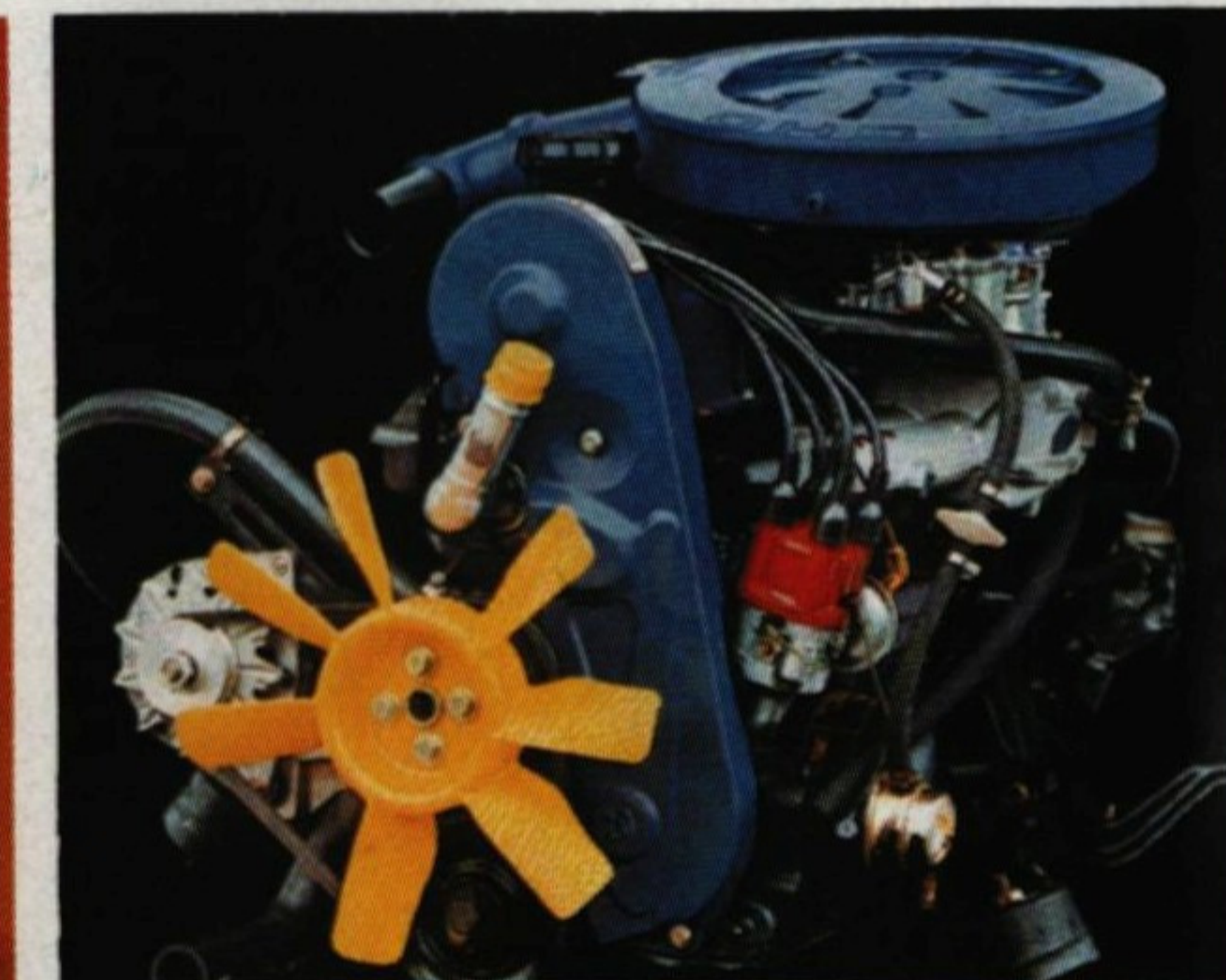
Das 3-Liter-V6-Triebwerk ▼
