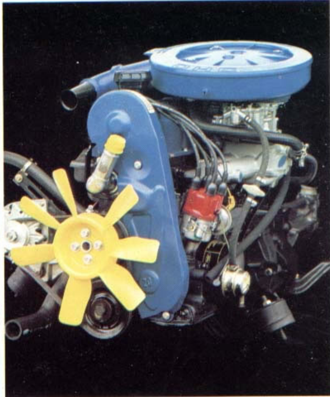
4-cylindret rækkemotor med overliggende knastaksel, 99 DIN HK ved 5000 o/min, drejningsmoment 15,4 kgm ved 4000 o/min, kompressionsforhold 9,2:1.
